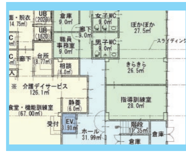
新会館の図面
